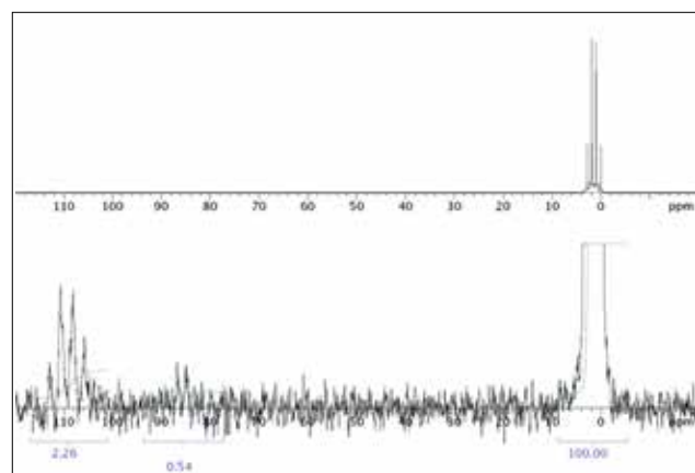
Рис. 6. 13 C спектр силикона после контакта с ПФД: спектр полностью (вверху), тот же спектр увеличенный (внизу) – видно пики ПФД в образце, что говорит о частичном растворении ПФД в силиконе
