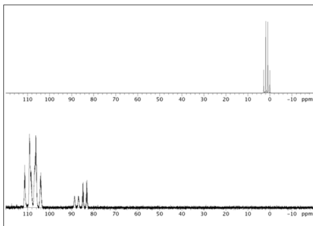
Рис. 5. 13 C спектры чистых силиконового масла (вверху) и ПФД (внизу)
