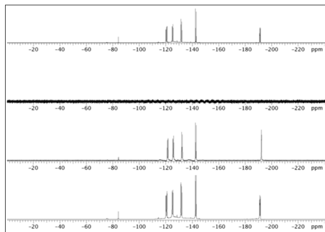
Рис. 4. 19 F спектры: 1 – чистый ПФД, 2 – чистое силиконовое масло, 3 – силиконовое масло после контакта веществ (содержит пики, соответствующие ПФД), 4 – ПФД после контакта веществ
