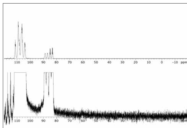
Рис. 7. 13 C спектр ПФД после контакта с силиконом: вверху спектр полностью, внизу тот же спектр увеличенный – видно отсутствие пиков силикона в образце, что говорит о том, что силикон в ПФД не растворяется. Данный спектр был получен усреднением 32 768 накоплений, остальные спектры получены усреднением 1024 накоплений
